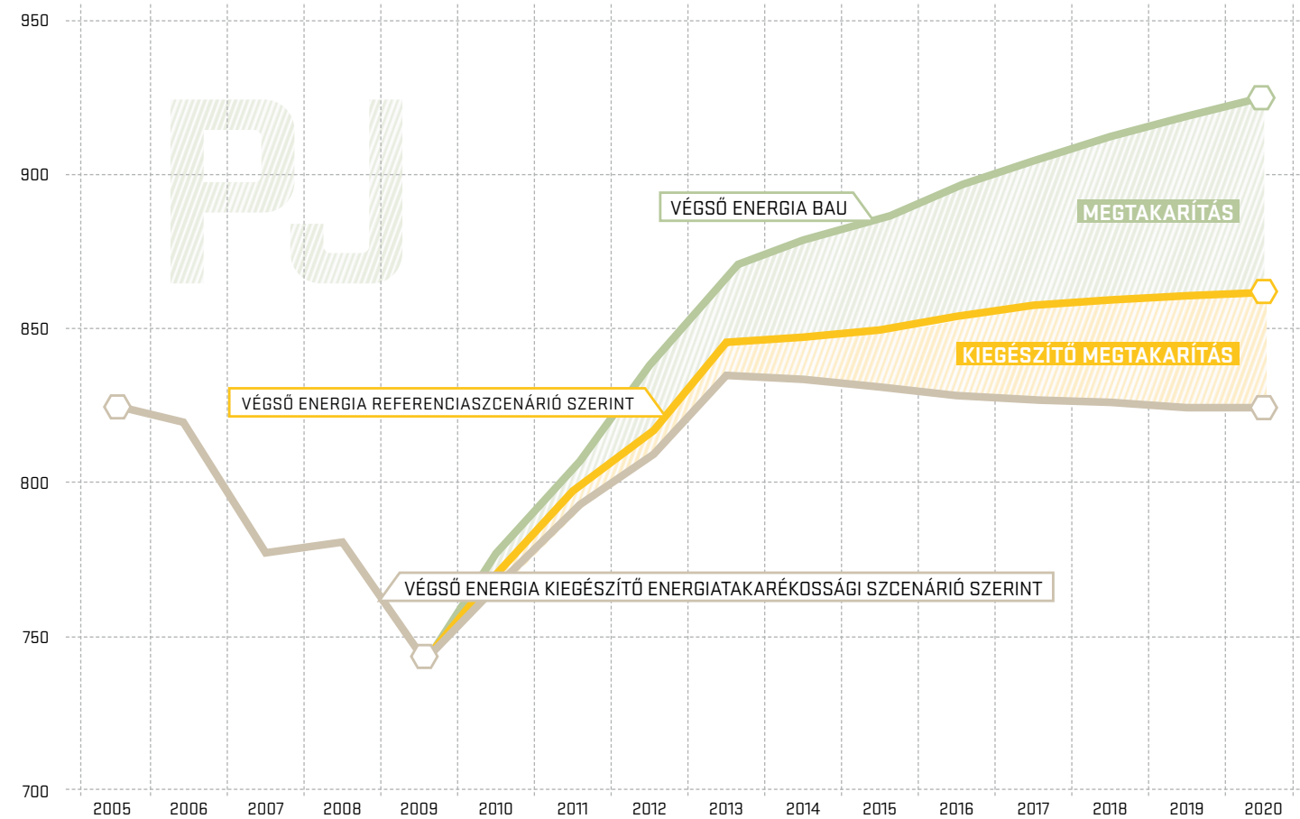
A végső energiafelhasználás scenáriói (PJ)
